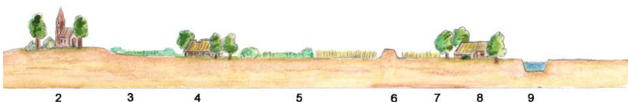
Een dwarsdoorsnede van de Vredewoldse situatie met betrekking tot de situatie na de commerciële turfgraverijen ten noorden van de Jonkersvaart in de negentiende eeuw: 1 = laagveenrivier, 2 = de primaire ontginningsas, 3 = tot kampen gedegenerende akkers, 4 = de secundaire bewoningsas, 5 = akkerboom, 6 = de leidijk, 7 = het afgegraven hoogveenpakket ten zuiden van de leidijk, 8 = boerderijen aan het Achterdiep, 9 = de Jonkersvaart.
